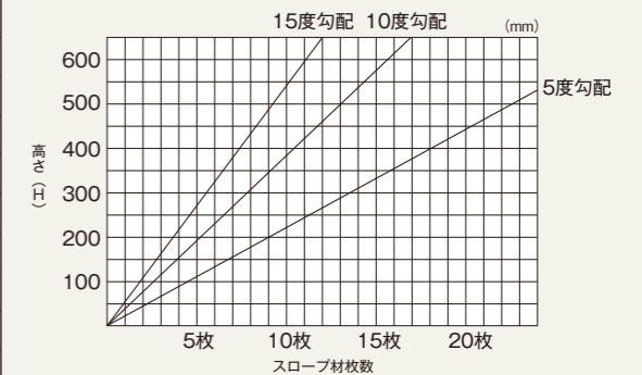
高さ勾配によるスロープ材枚数の導き出す表
